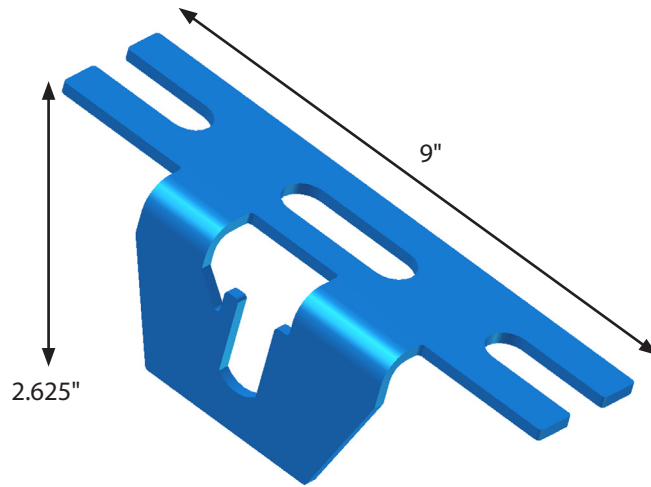
915BPSR DWG #351
