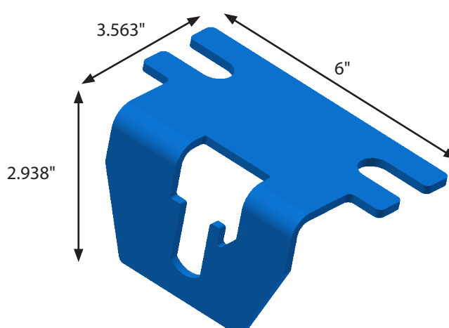
620CIR DWG #719
